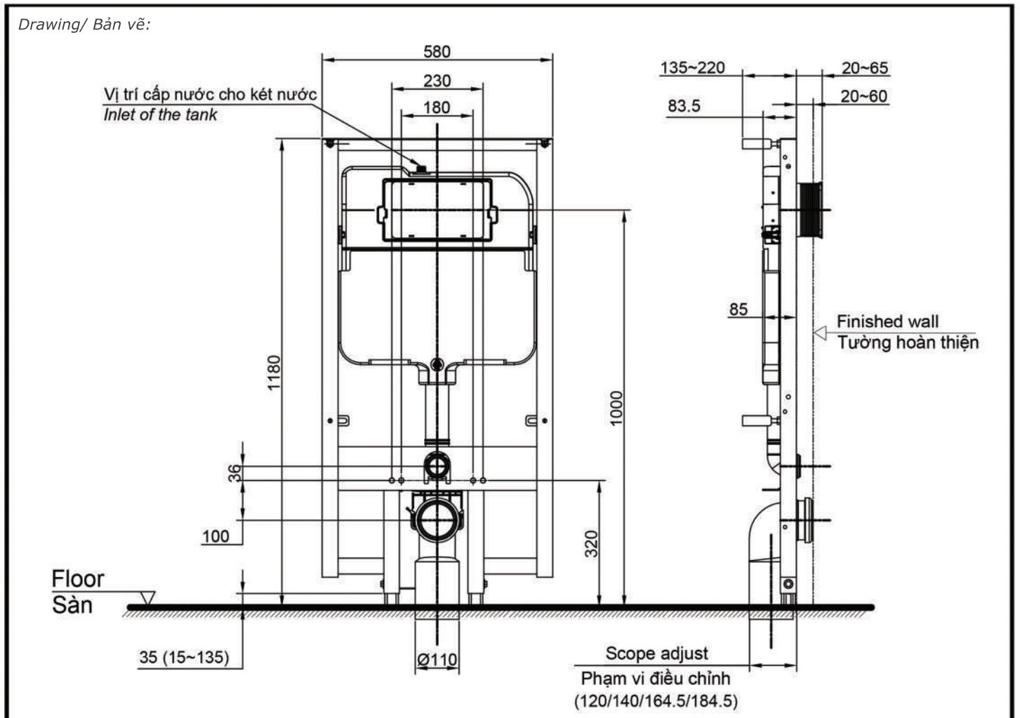
Concealed tank Kết nước âm tường
